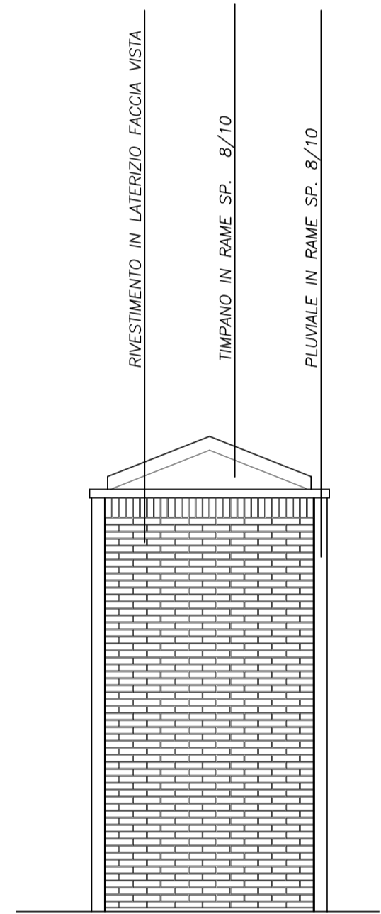
RETRO
