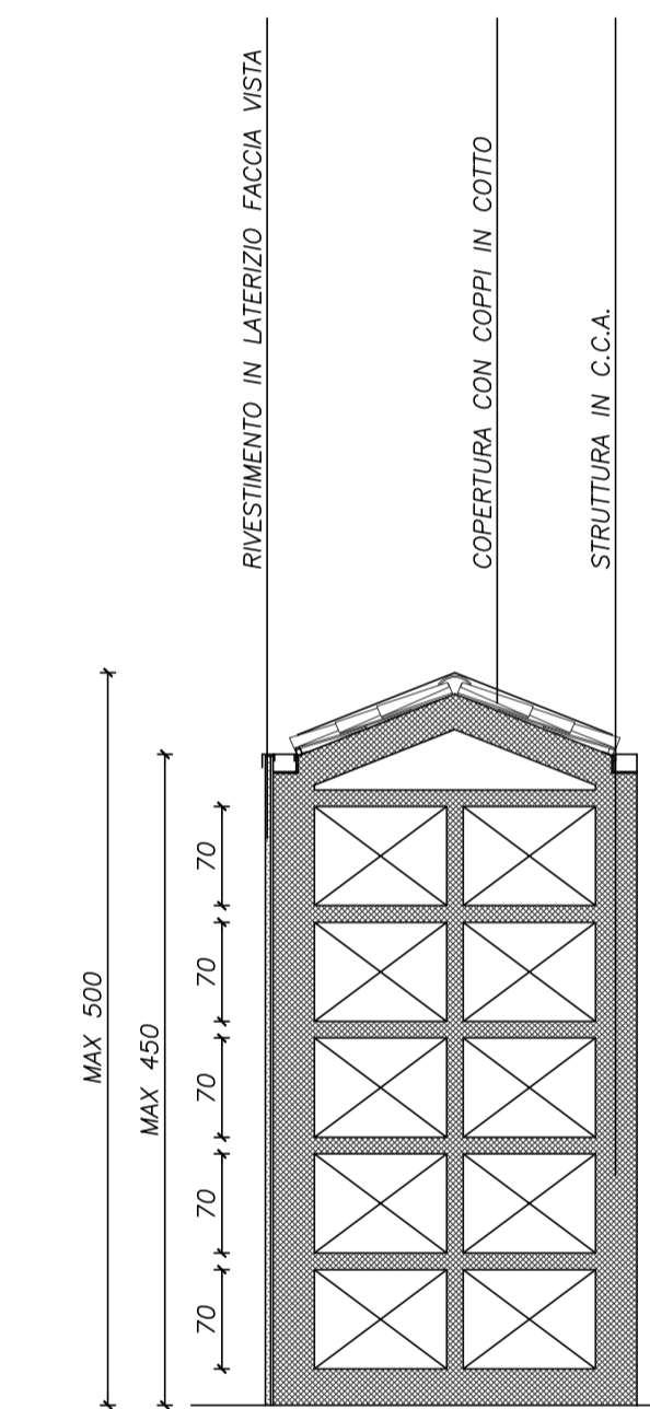
SEZIONE A-A
