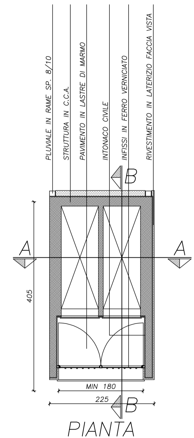
PIANTA
