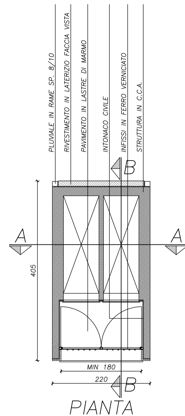
PIANTA
