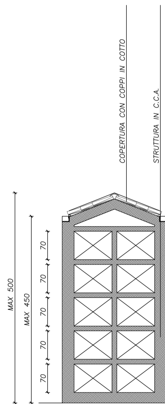
SEZIONE A-A
