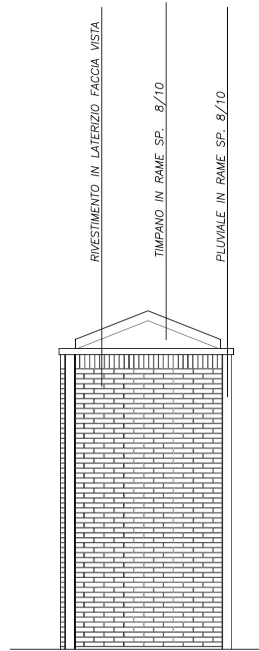
RETRO
